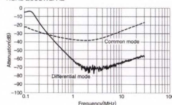
RSAL-2003WL/AL
