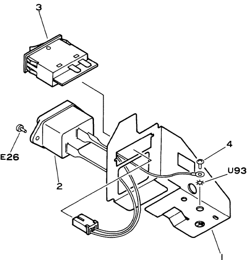
FIGURE 110 MAIN SWITCH ASSEMBLY メイン・スイッチ部
