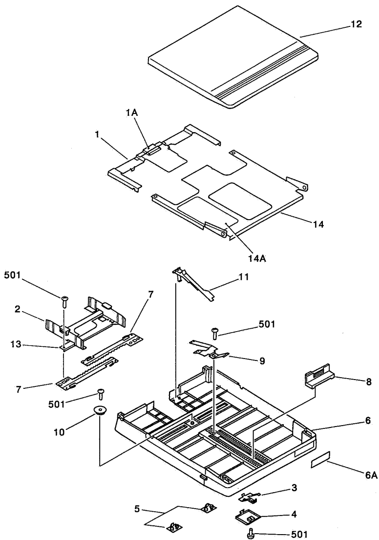
FIGURE 304 CASSETTE (X1) カセット (X1)
