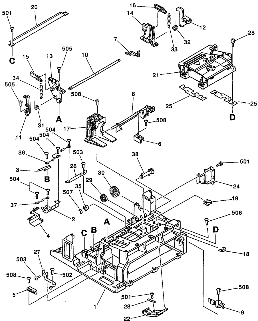
FIGURE 320 MAIN BODY BLOCK ASS'Y 本体ブロック部
