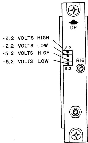
Figure 3-9. PL Module
